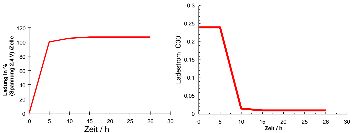
Abb.2 Zyklischer Betrieb
