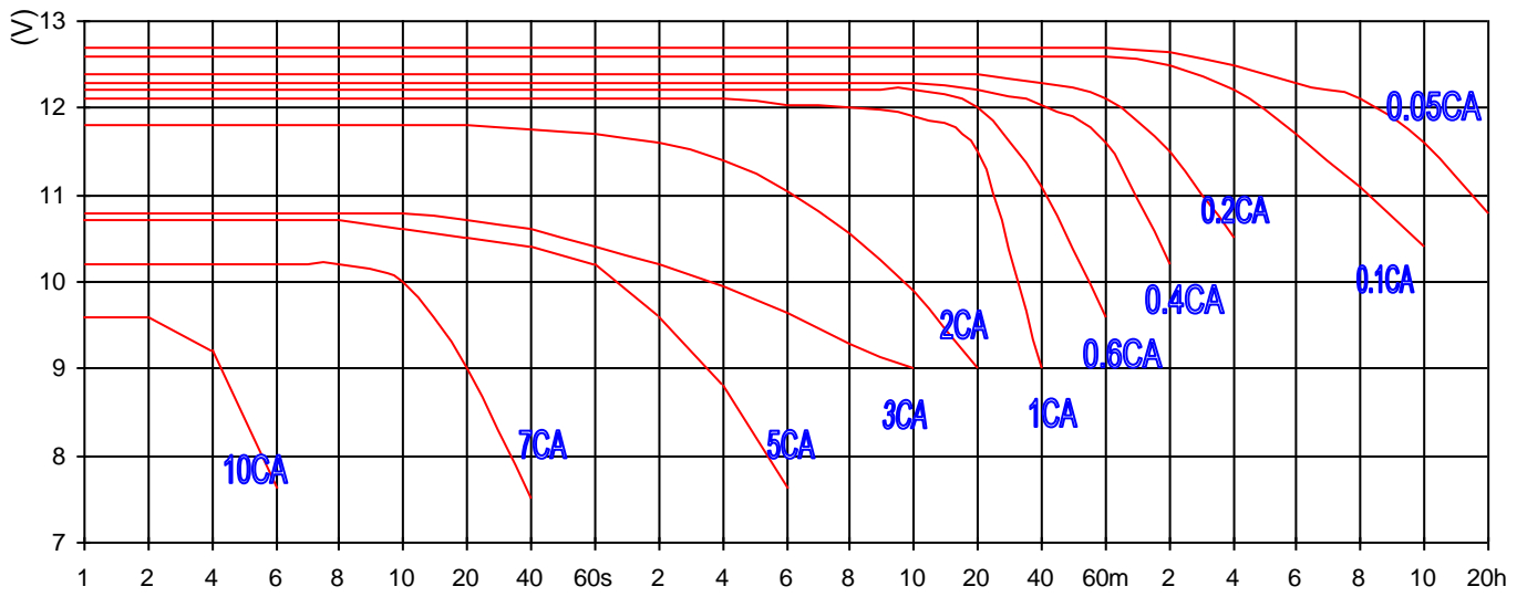
Abb.3: Entlade-Kennlinien (C=20)
